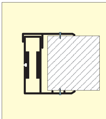
4. PK4 alumiini Rakenne 80 mm
