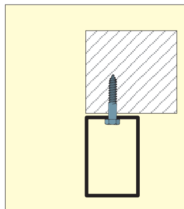
6. PK6 Neliökarmi teräs/alum 40x60 mm
