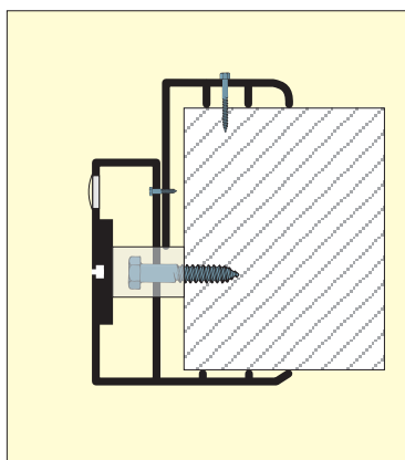
2. PK2 alumiini Rakenne 70-130 mm
