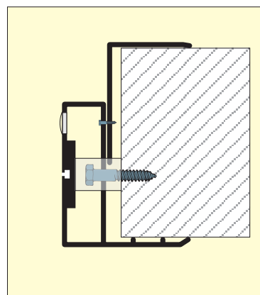
3. PK3 alumiini Rakenne 130-170 mm
