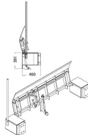
Kärkilevy käyttöasennossa auton lavalla
